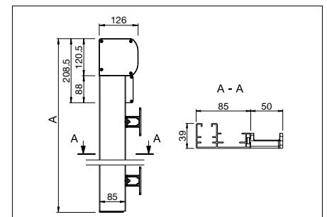
Wandmontage mit Befestigungshalter FS-602-1 A = Total Höhe
