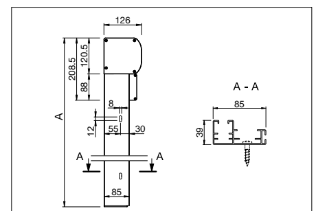
Laibungsmontage A = Total Breite
