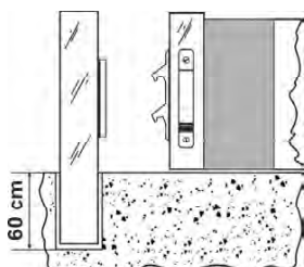
Bodenhülseenansicht
