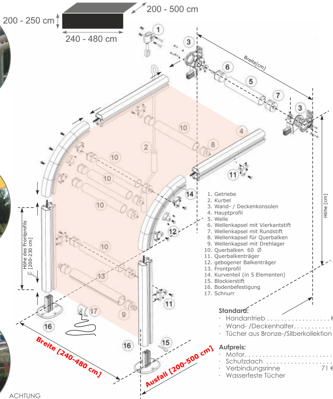
Verbindungsrinne (Option)
